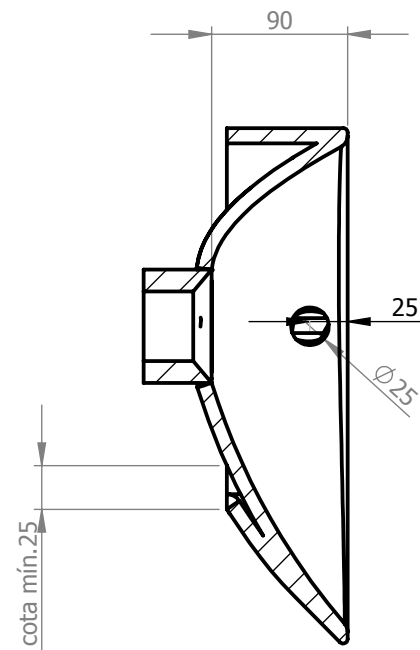
SECCIÓN B-B
