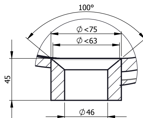
DETALLE H ESCALA 2 : 5
